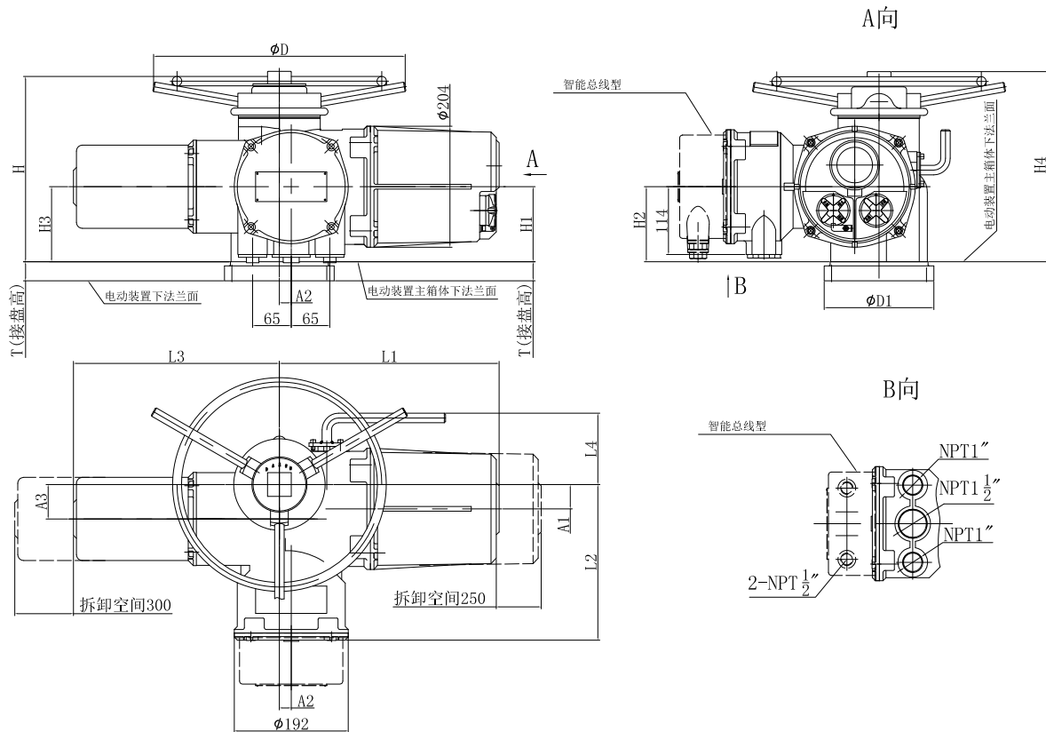
IMC15~60系列外形尺寸
